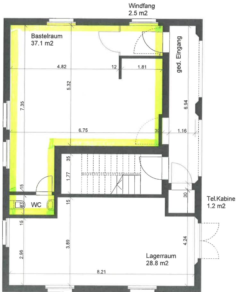
Erdgeschoss 1:100
